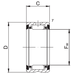
RNA49UU, RNA69UU (Fw ≤ 35)
