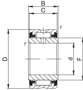
NA49UU,NA69UU(d ≤ 30)
