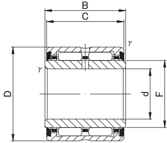
NA69UU
